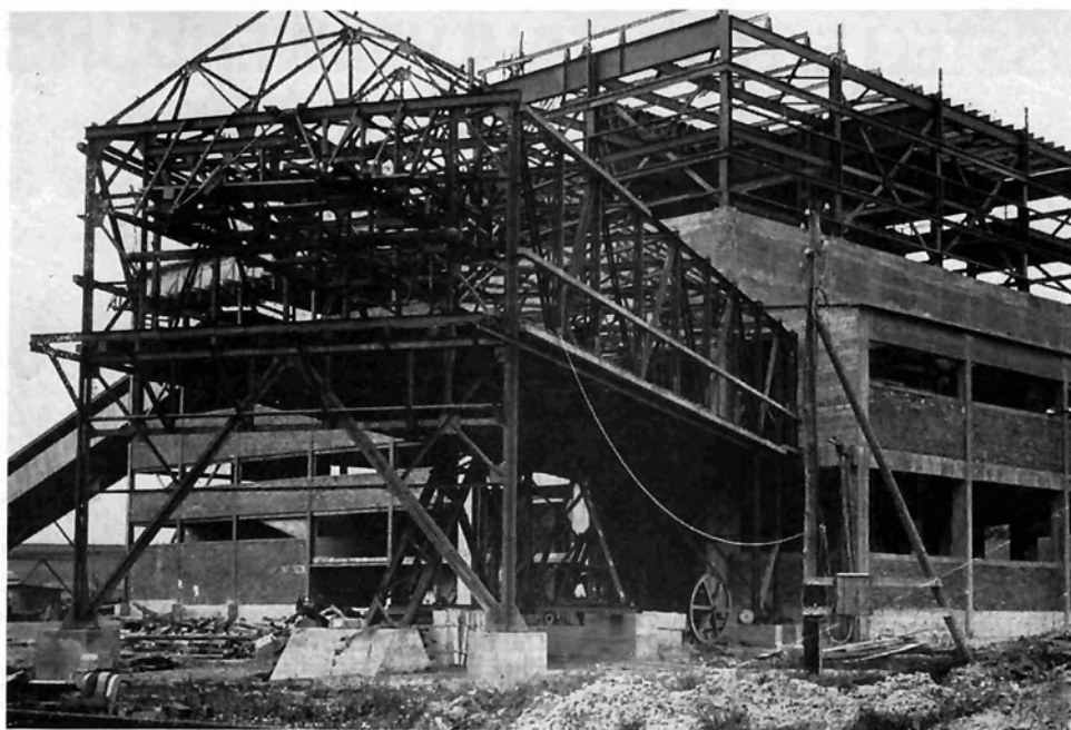
Stahlkonstruktion für Hallenbau
