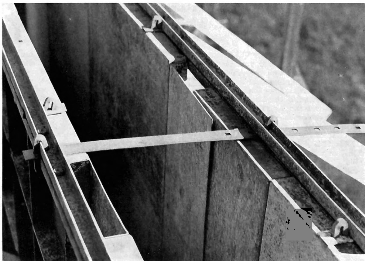
Bild 3: Befestigungselemente und Schleifbleche der Stahl-Bauschalung
