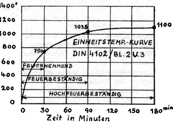
Bild 3: Einheitstemperaturkurven Fig. 3: Specific temperature curves
